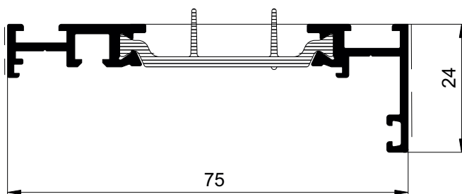
Притвор порога 24
