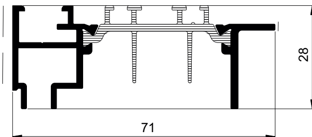
Профиль подставочный 28
